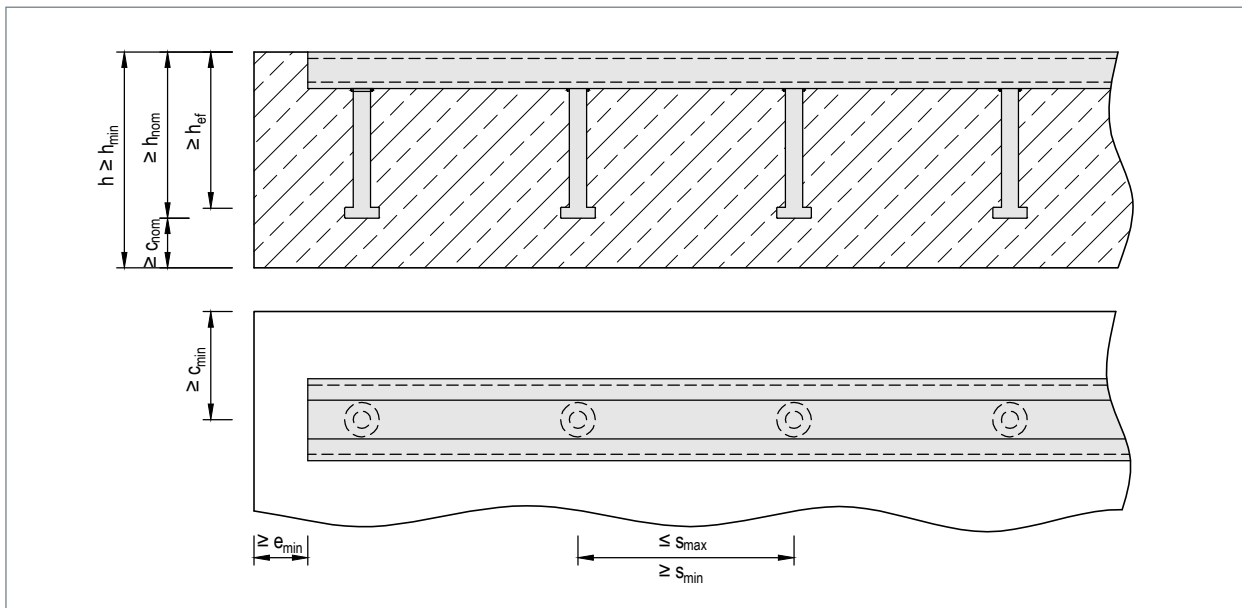
▲ MBA-CE: Indbygningstilstand
